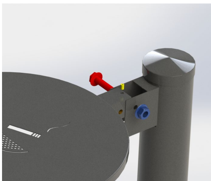
M6x45 TBEI
